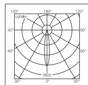
HIT-CE 35w Medium
