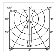
HIT-CE 70w Medium
