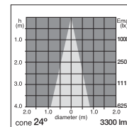
35w HI-PAR 36 24° lamp
