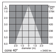
35w HIT-TC-CE
