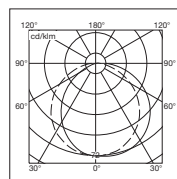
38w 3 Bar Grille
