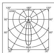
HIT-CE 70w Spot
