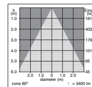
cone 60° 70w WB
