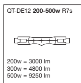
ULOR = 0.82 4041643
