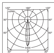
HIT-CE 35w Spot
