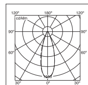
HIT-CE 35w Flood
