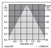
cone 60° 35w WB
