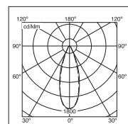
HIT-CE 70w Flood
